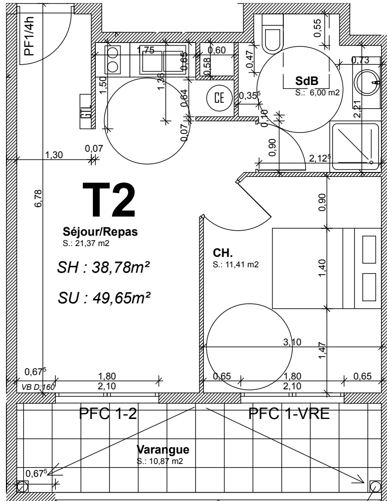
PLAN ET FACADE POUR REPERAGE
