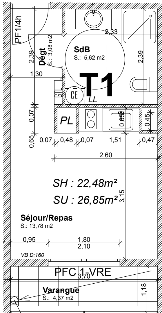
PLAN ET FACADE POUR REPERAGE
