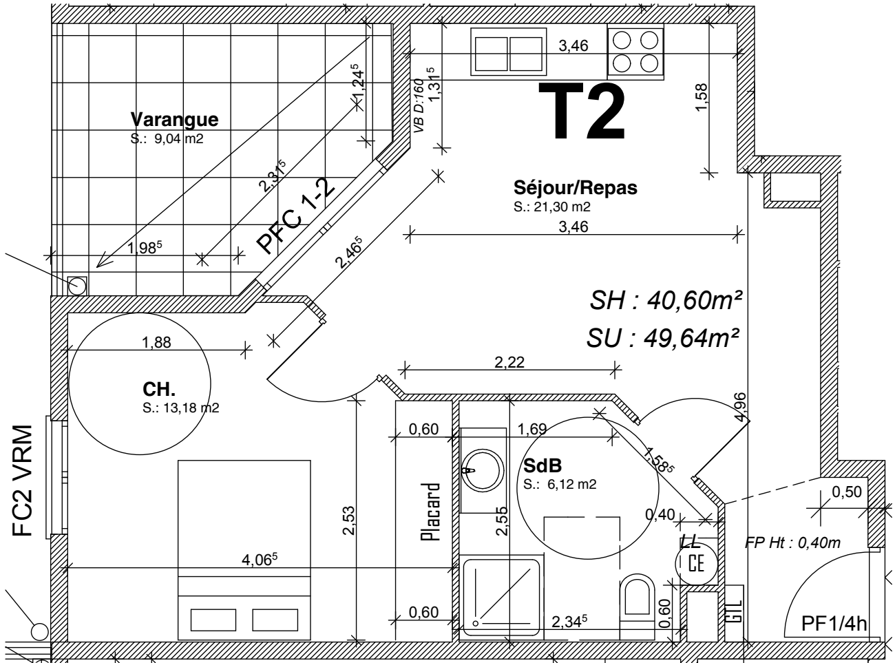
PLAN ET FACADE POUR REPERAGE
